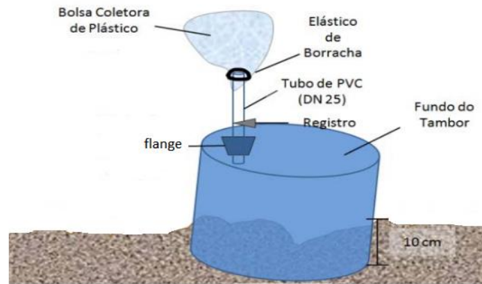
Figura 5 - Seepage meter. (Adaptado de Kern, 2018) superfície da água
