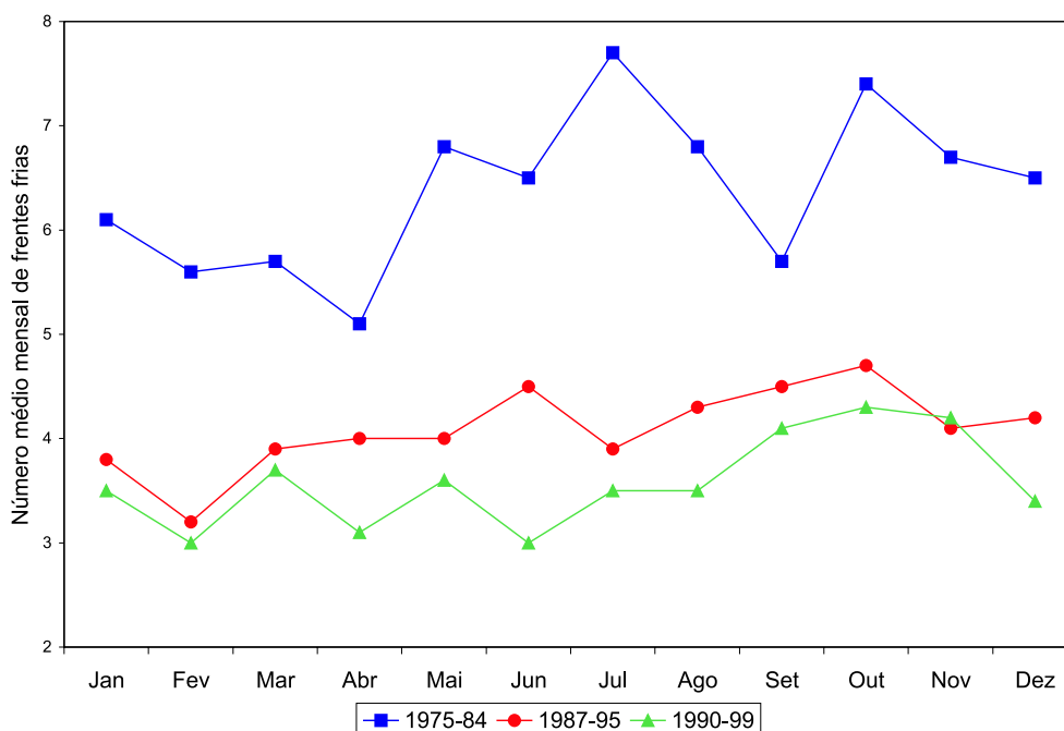
Figura 4 – Número médio mensal de frentes frias em diferentes estudos no litoral de Santa Catarina.
